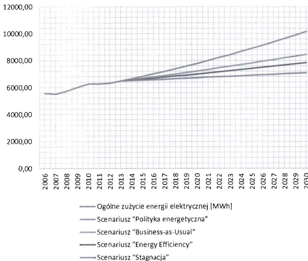
Rysunek 19. Symulacja zapotrzebowania na energię elektryczną [MWh] wg założonych scenariuszy do roku 2030.
